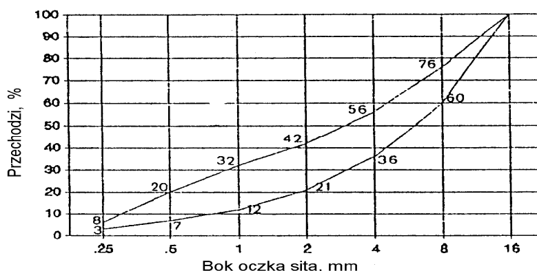
Rysunek 1. Krzywe graniczne uziarnienia kruszywa do betonu
