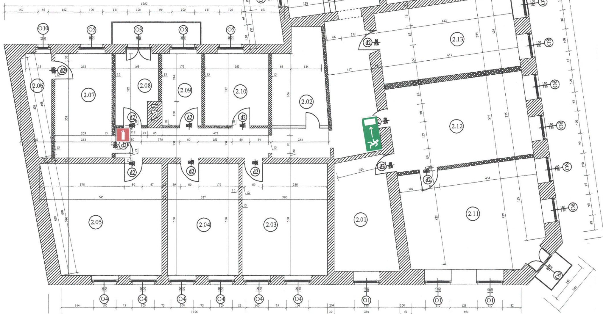
RZUT I PIĘTRO STAN ISTNIEJĄCY, 1:100
